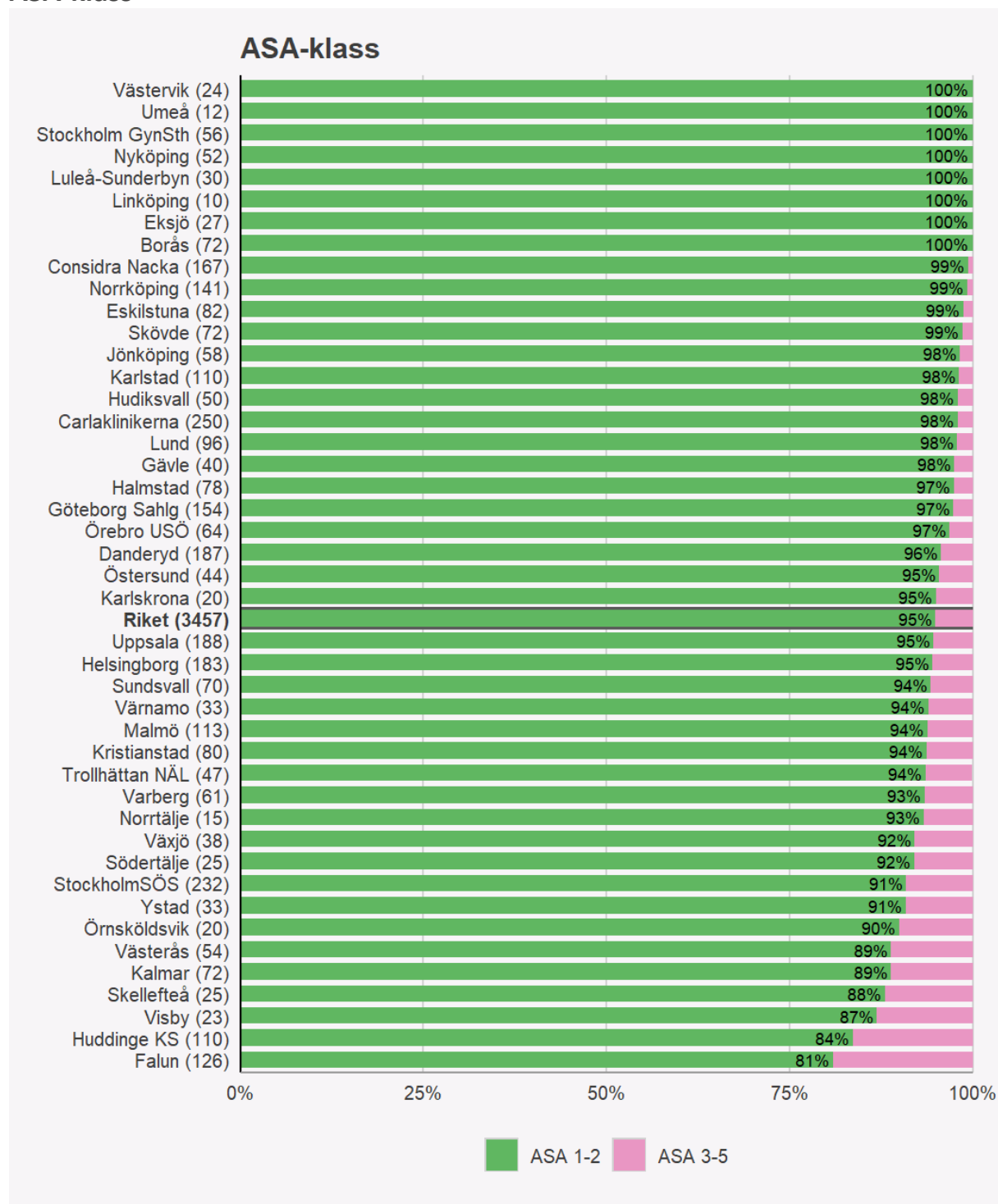
Figur 4. ASA-klass.
